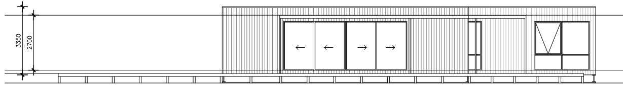
elevation 1
