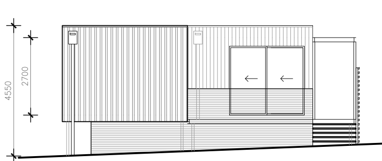
elevation 02
