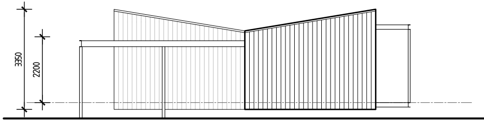
elevation 02
