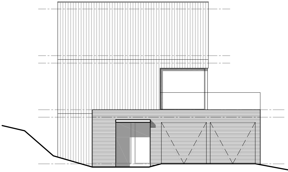
elevation 01
