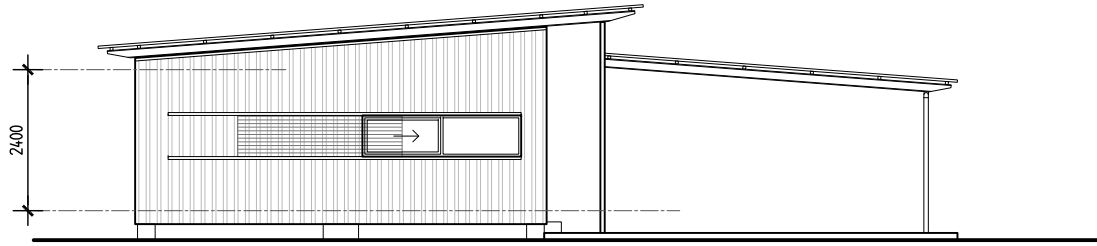
elevation 01
